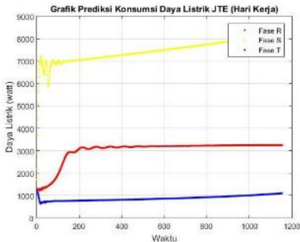
Gambar 9. Prediksi Kebutuhan Daya Listrik Tiap Fase pada hari kerja di Gedung Teknik Elektro Unila Pada Bulan Juni 2018
