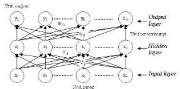
Gambar 2. Arsitektur Backpropagation
