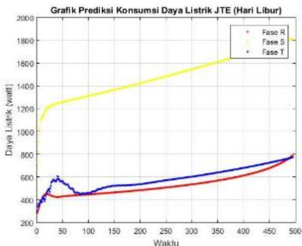
Gambar 10. Prediksi Kebutuhan Daya Listrik Tiap Fase pada hari libur di Gedung Teknik Elektro Unila Pada Bulan Juni 2018
