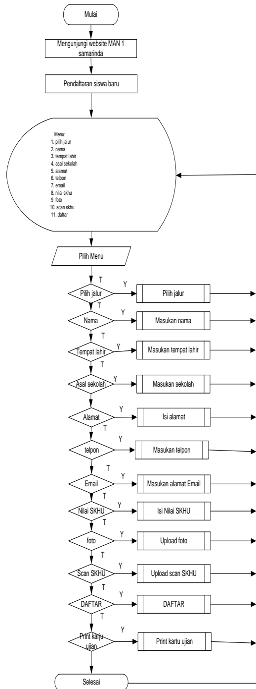
Gambar 5. Flowchart pendaftaran siswa baru
